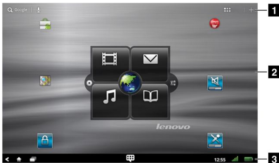
Obrázek 3. Obrazovka Domů
