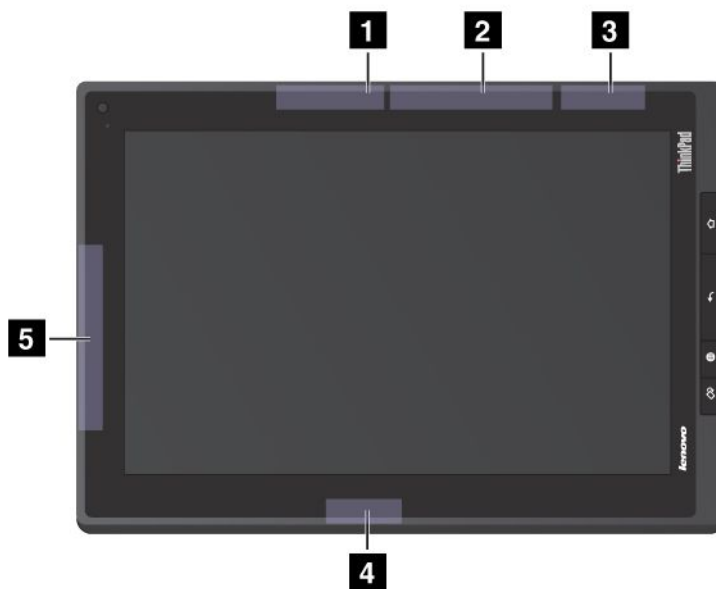
Obrázek 17. Umístění bezdrátových antén UltraConnect
